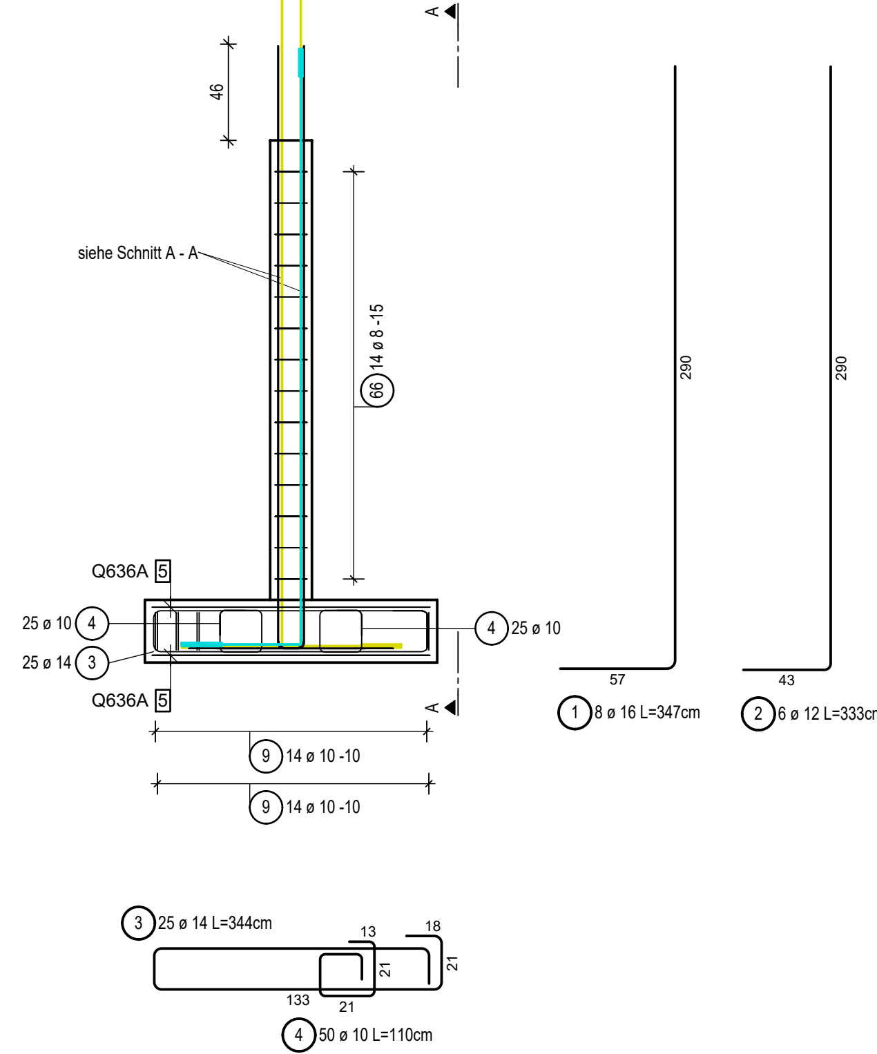
Schnitt 1 - 1
