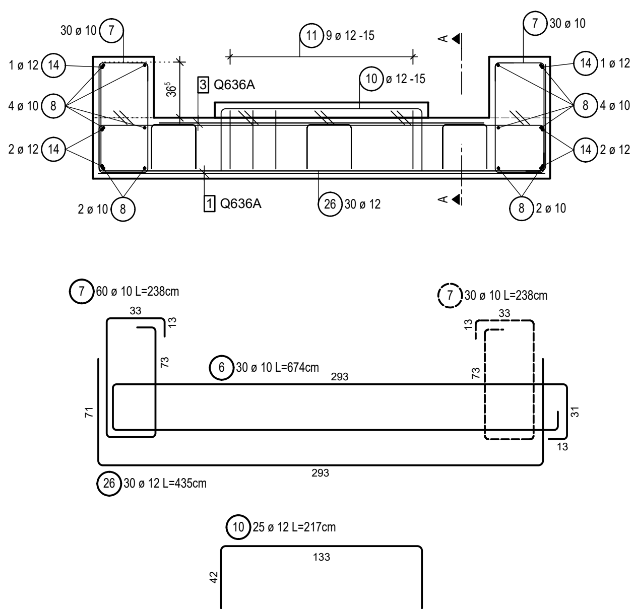
Schnitt 1 - 1
